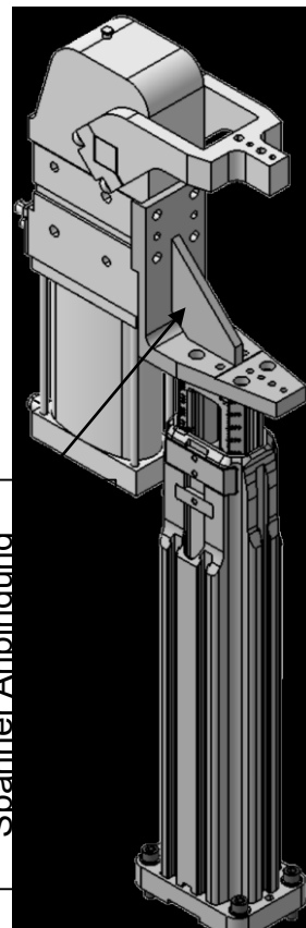
Spanner Anbindung Größe/Size 80 Auf Anfrage/on request
