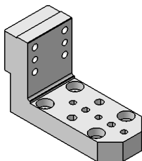
Spanner Anbindung/ Clamp Connection Größe/Size 40 1346000
