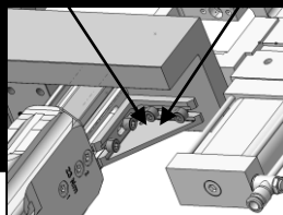
Verstärkungswinkel /Reinforcemen
