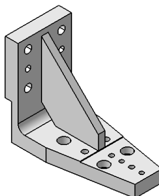
Spanner Anbindung/ Clamp Connection Größe/Size 80 Auf Anfrage/On Request
