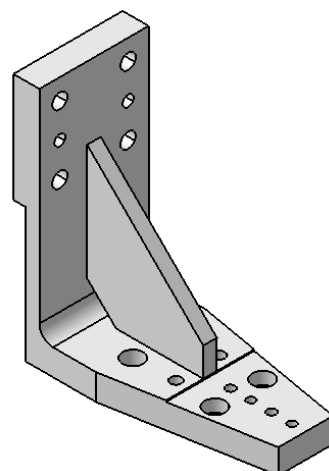
Spanner Anbindung/ Clamp Connection Größe/Size 80 Auf Anfrage/On Request
