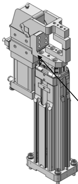
Spanner Anbindung Größe/Size 50 - 63 1346001
