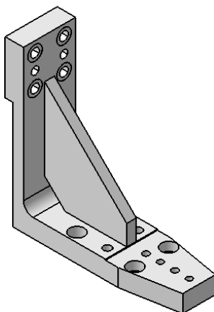
Spanner Anbindung/ Clamp Connection Größe/Size 50 - 63 Auf Anfrage/On Request
