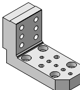
Spanner Anbindung/ Clamp Connection Größe/Size 50 - 63 1346001
