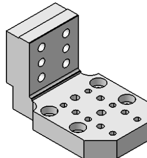
Spanner Anbindung/ Clamp Connection Größe/Size 50 – 63 quer/cross 1346002
